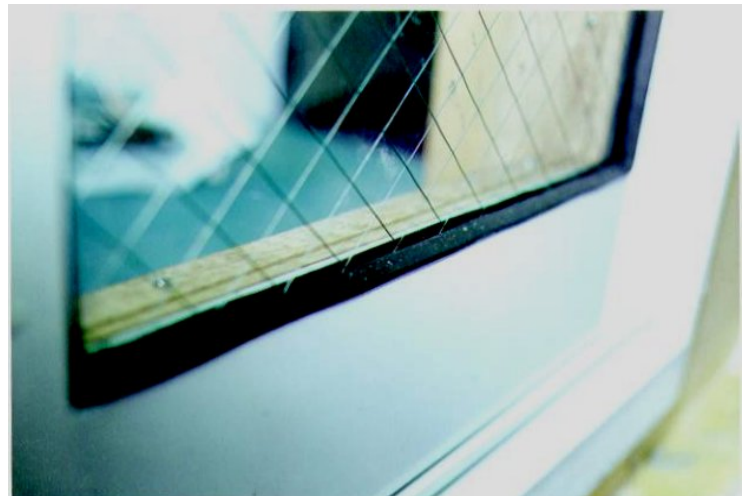
試験前(ガスケット部拡大)
